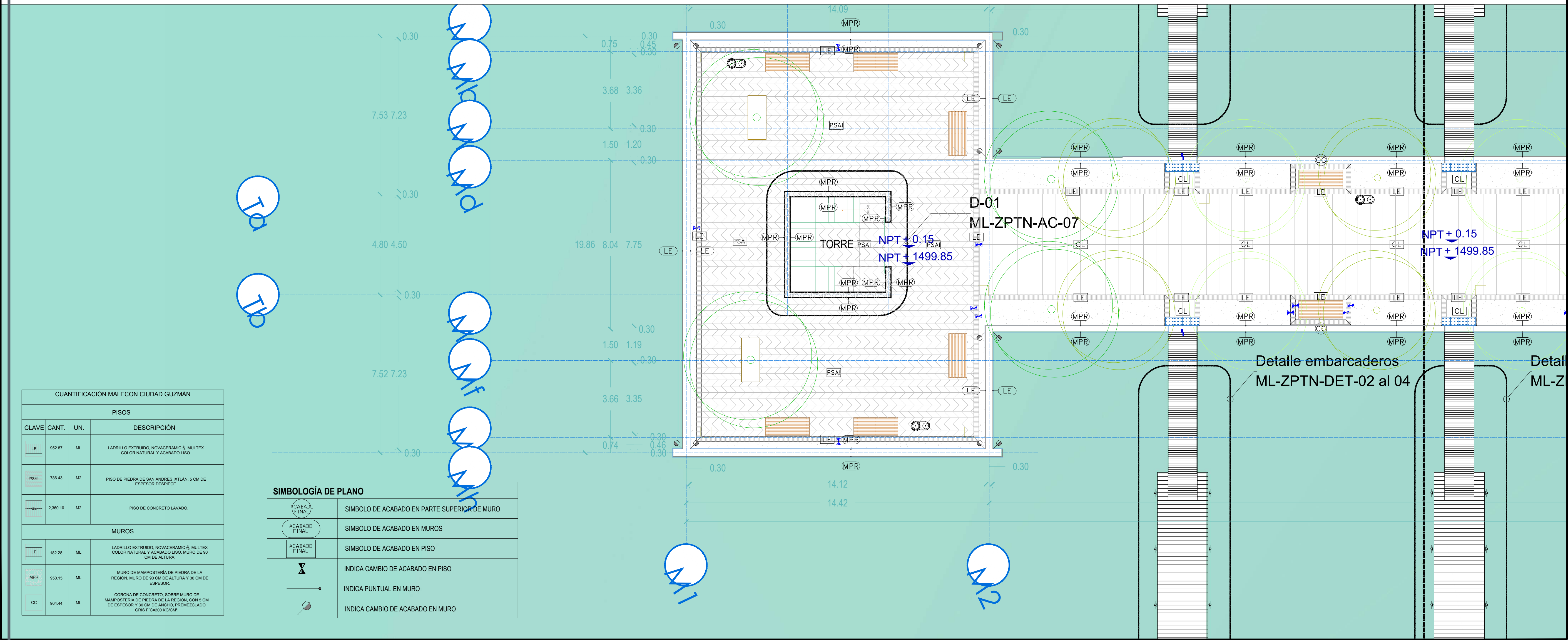
01 PLANO DE ACABADOS TRAMO 1 ML-ZPTN-AC-01 1:100
