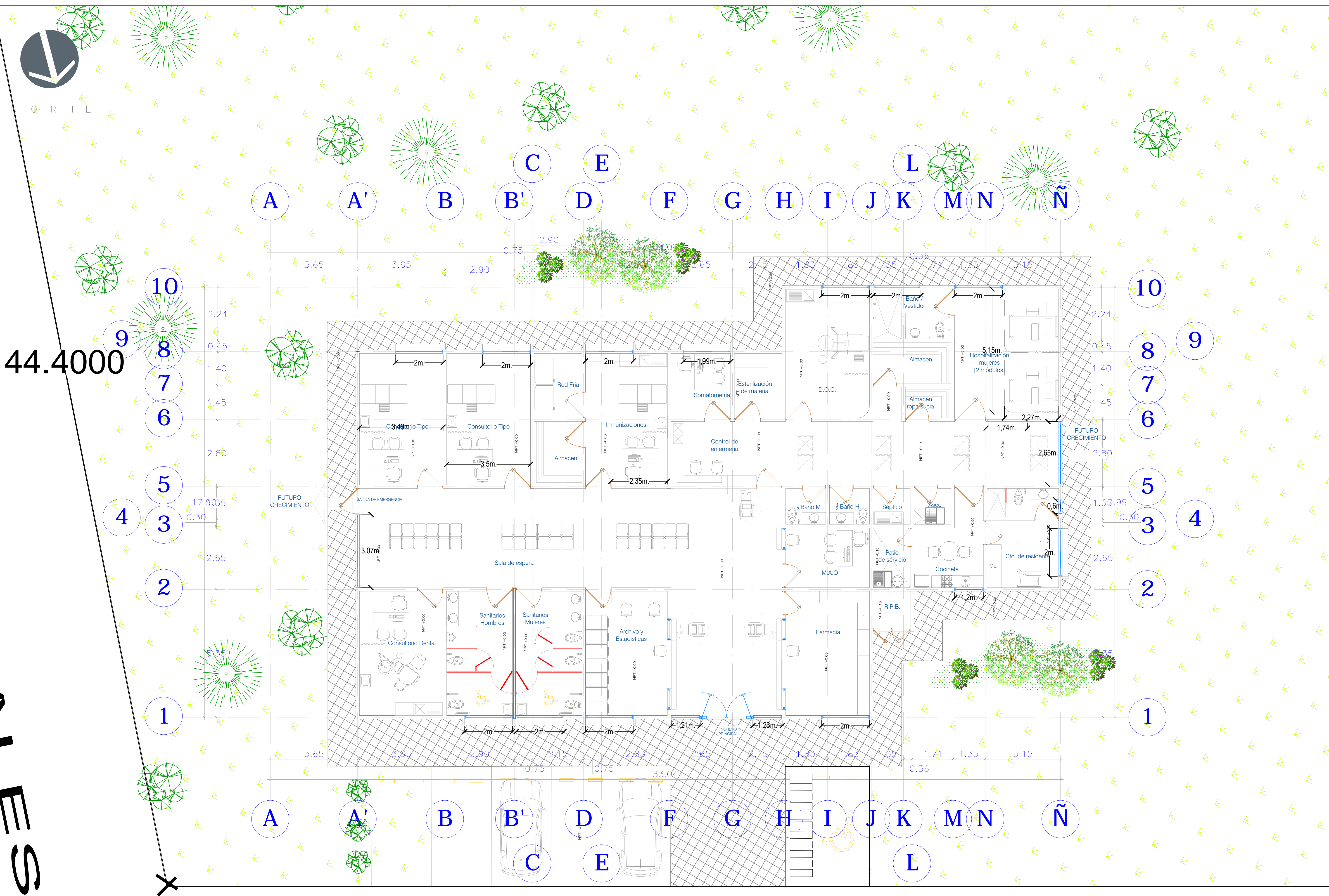
01 PLANTA ARQUITECTÓNICA 1:50
