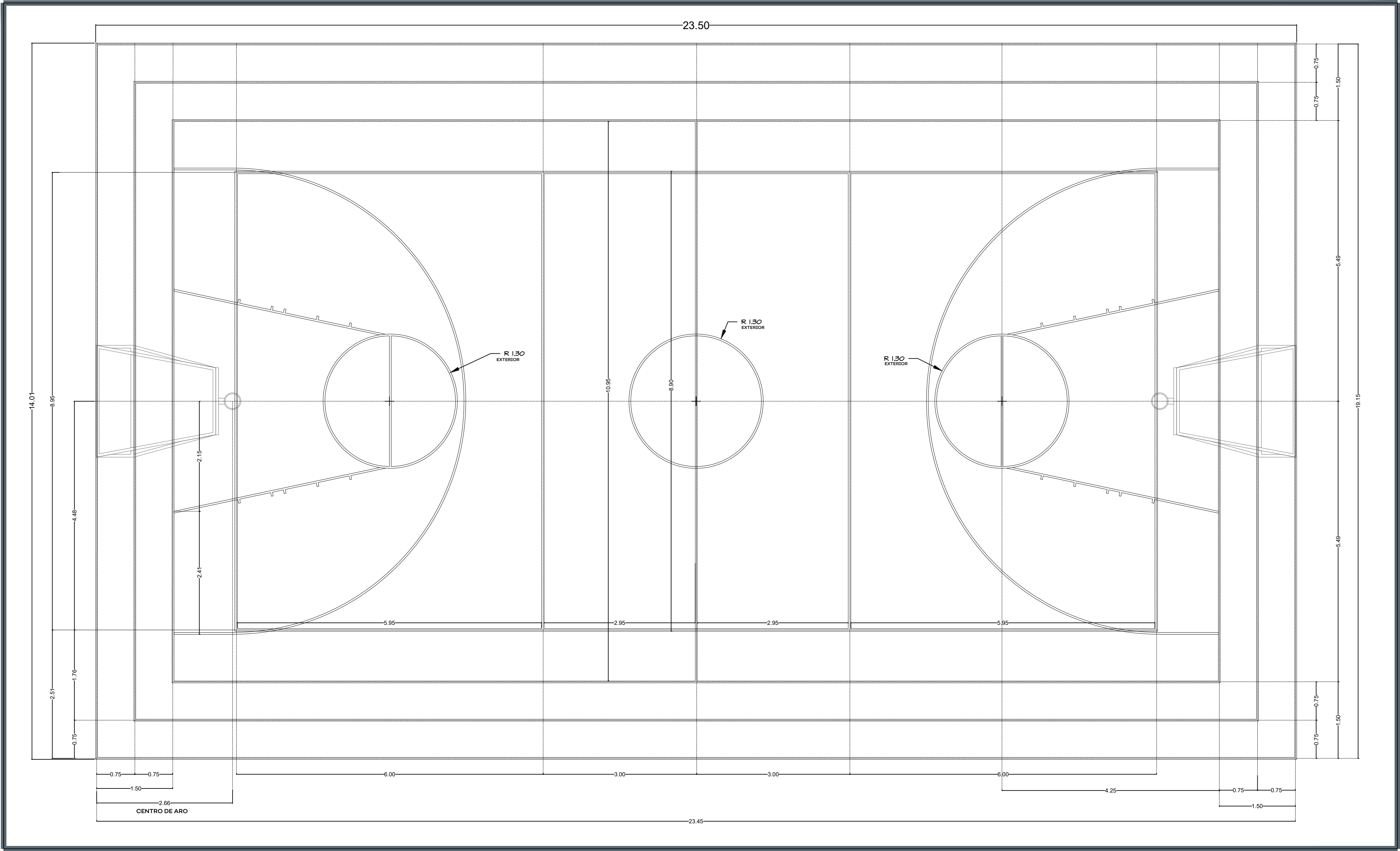
01 BALIZAMIENTO- CANCHA DE USOS MÚLTIPLES 1:100
